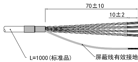
电缆连接
