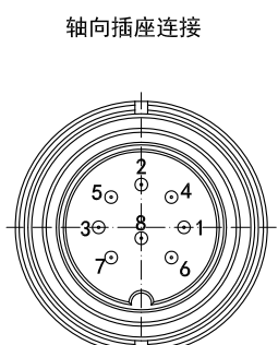
M16-8DIN针公座引脚分配图
