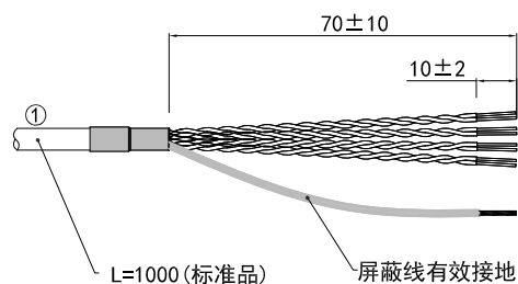
径向电缆连接
