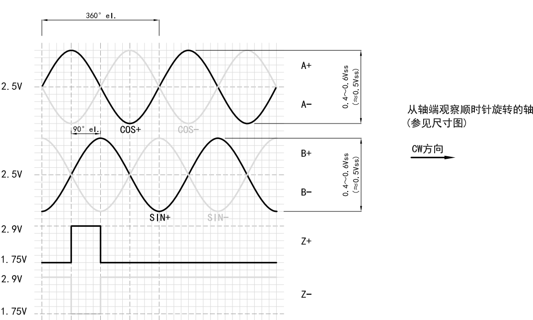
4.4 差分生成前的正弦/余弦增量信号
